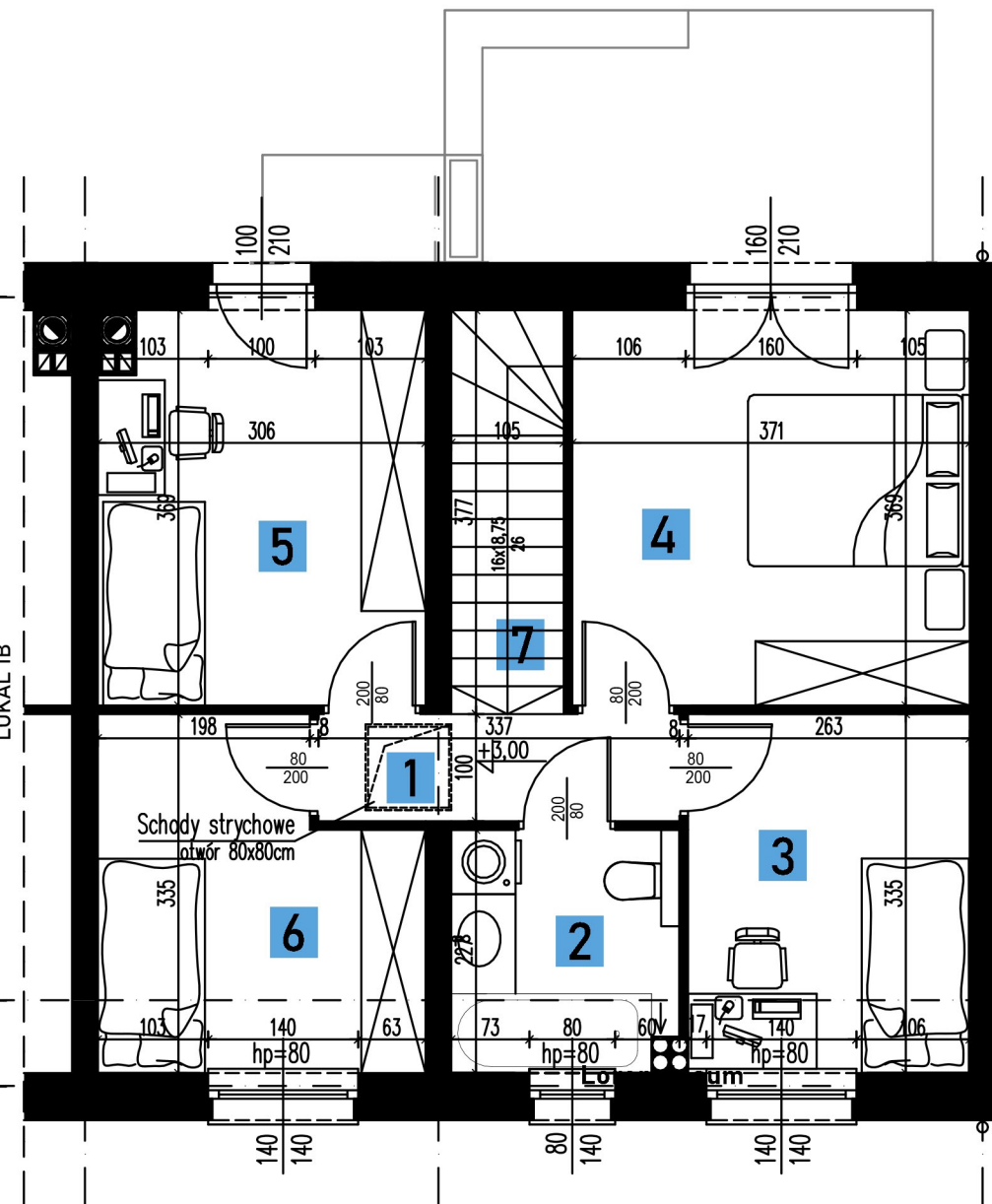
RZUT PIĘTRA
