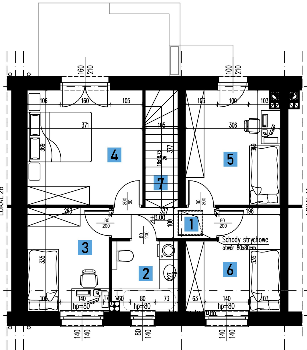
RZUT PIĘTRA
