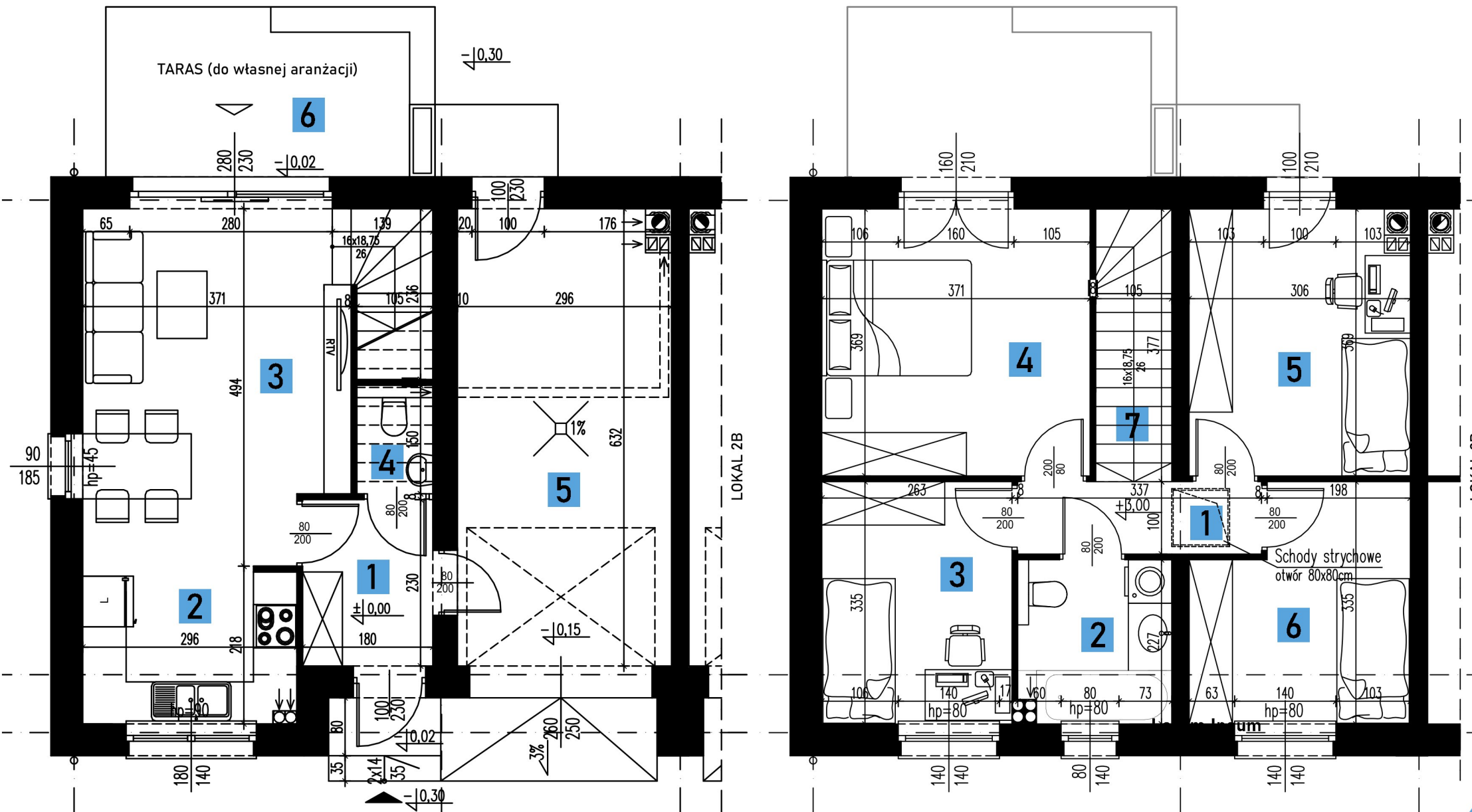
RZUT PARTERU
