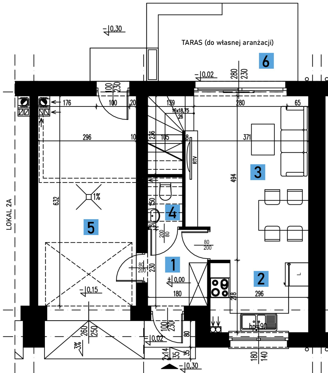
RZUT PARTERU
