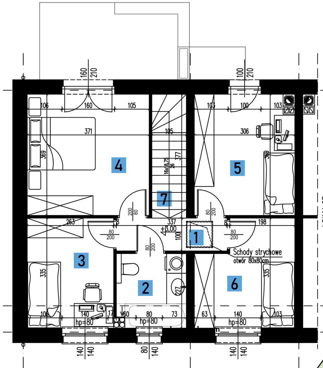
RZUT PIĘTRA
