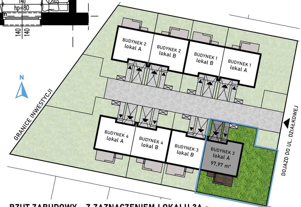
RZUT ZABUDOWY - Z ZAZNACZENIEM LOKALU 3A
