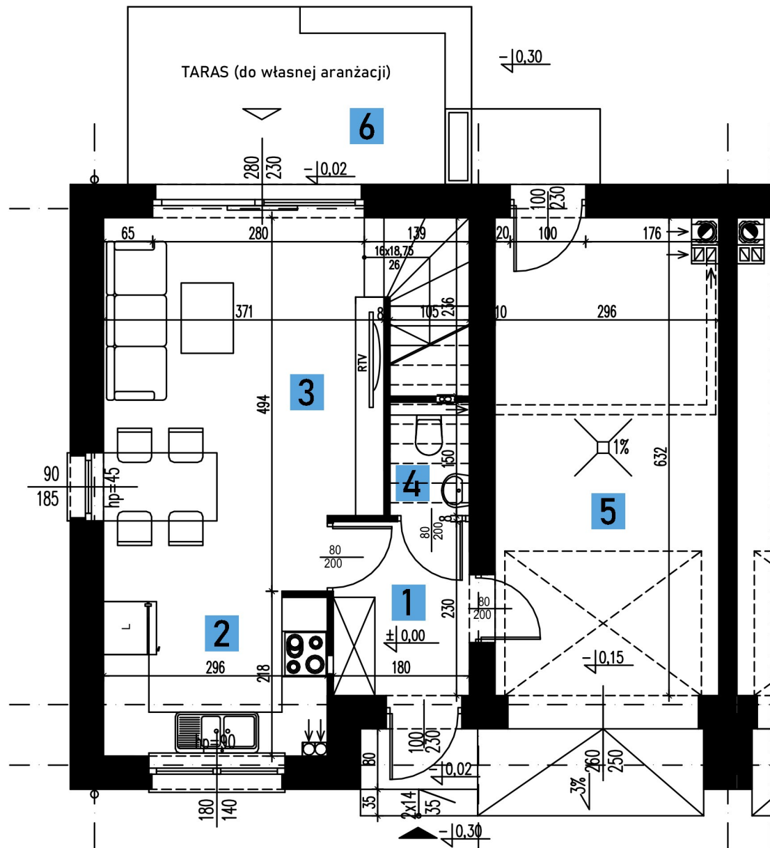
RZUT PARTERU
