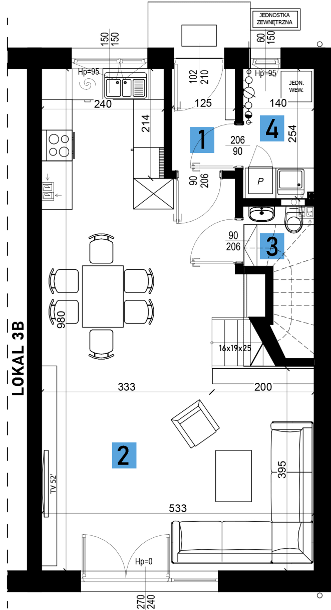
RZUT PARTERU
