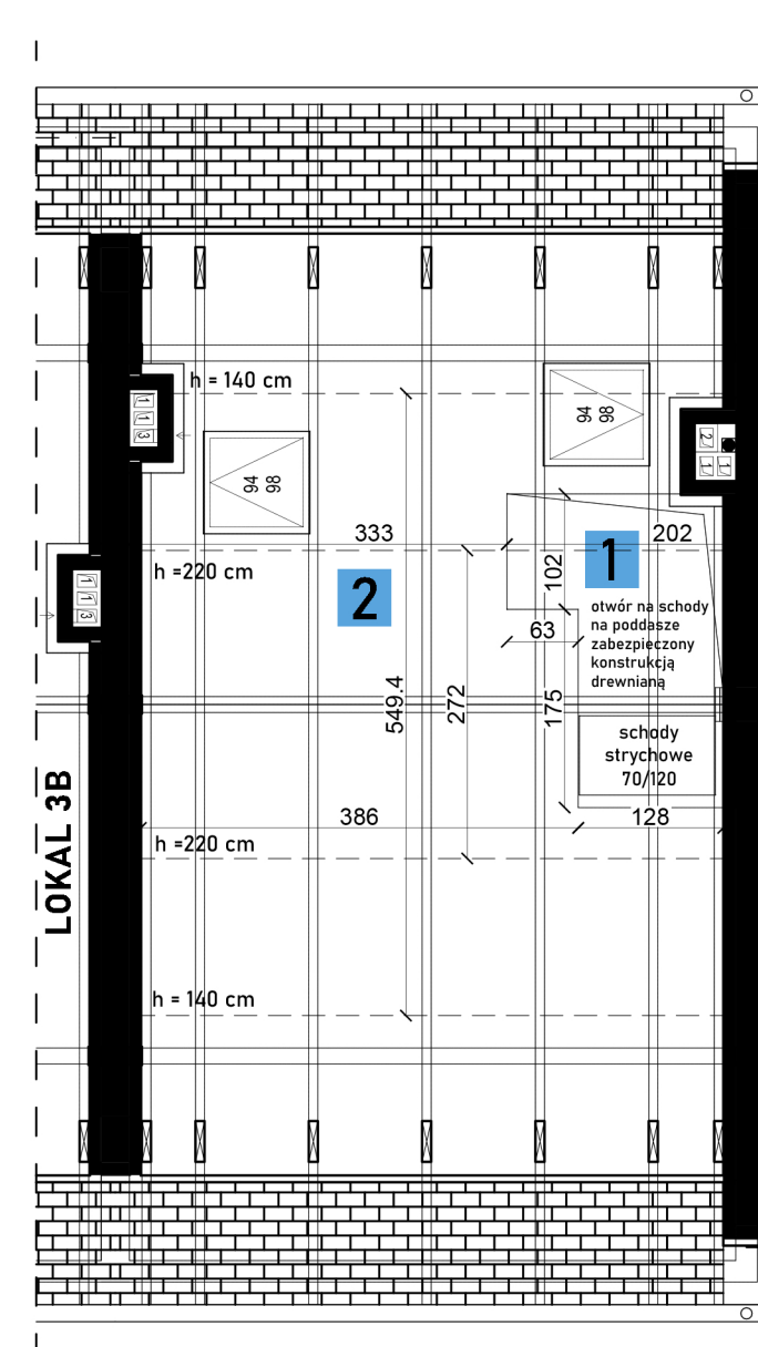
RZUT PODDASZA NIEUŻYTKOWEGO
